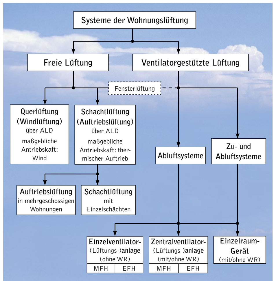
Überblick der Wohnungslüftungssysteme gemäß ihrer Wirkungsprinzipien
