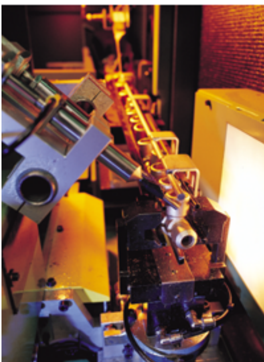
Membran-Sicherheitsventile auf der Transfairstation mit angegliederter Qualitätsüberwachung
