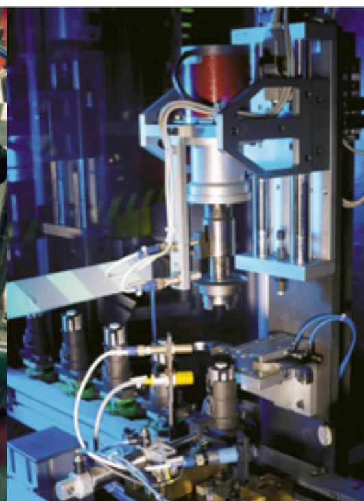
Die Positionskontrolle erfolgt auf den automatischen Fertigungsinseln durch Robot-Stationen
