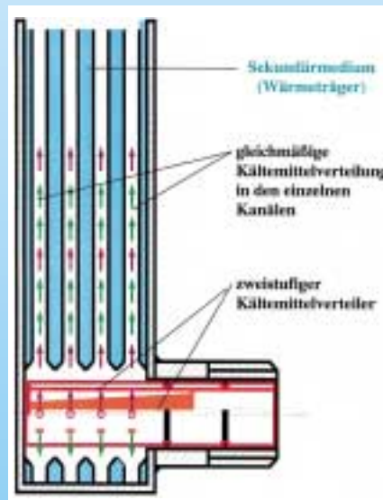
Erhöhung der Leistungszahl durch Plattenverdampfer mit Kältemittelverteiler und abgestimmtem Expansionsventil
